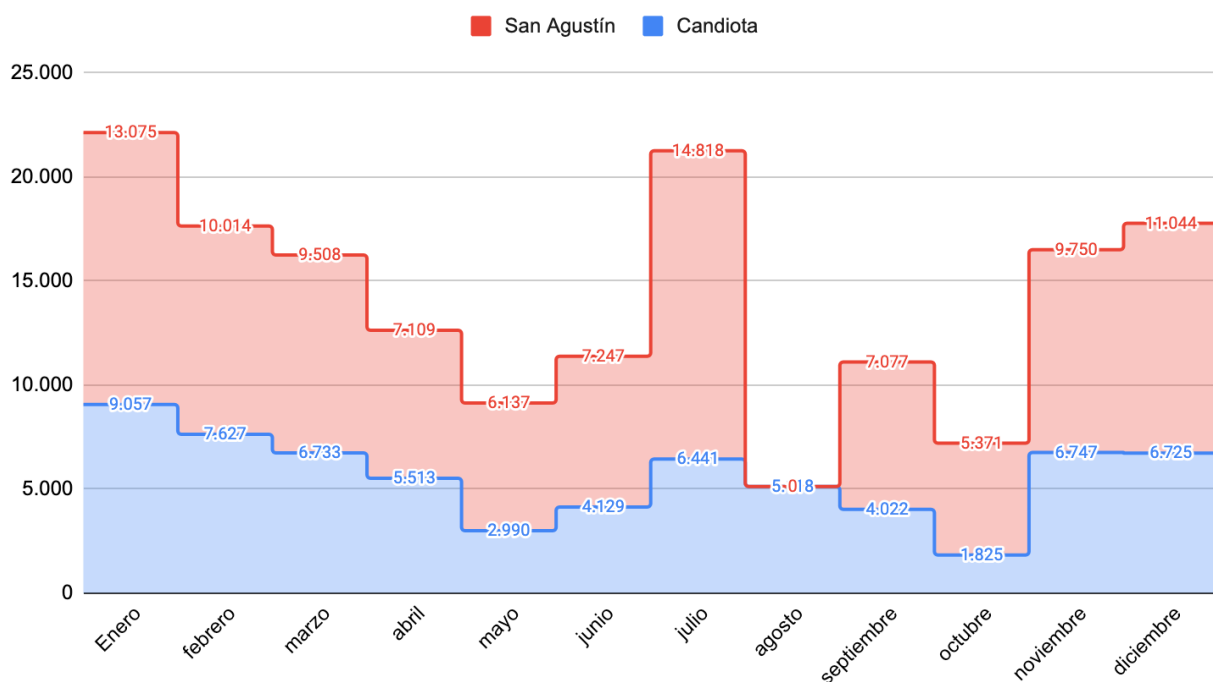
Consumos eléctricos por periodos de facturación (kWh)
